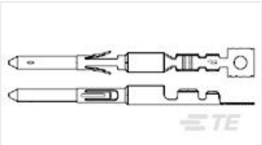
TE Part #66728-5 CIRC DIN PIN CONTACT,LP
