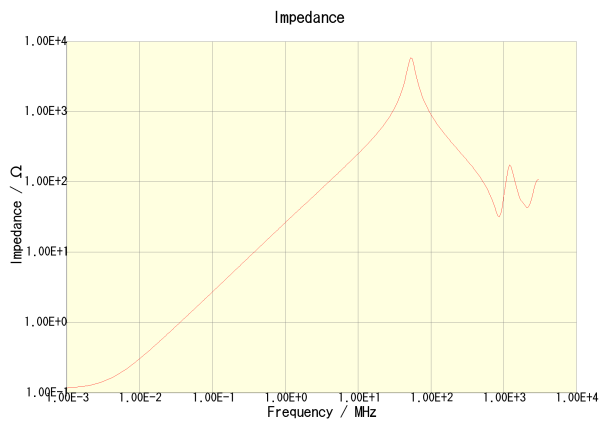
VLS3015ET-4R7M
