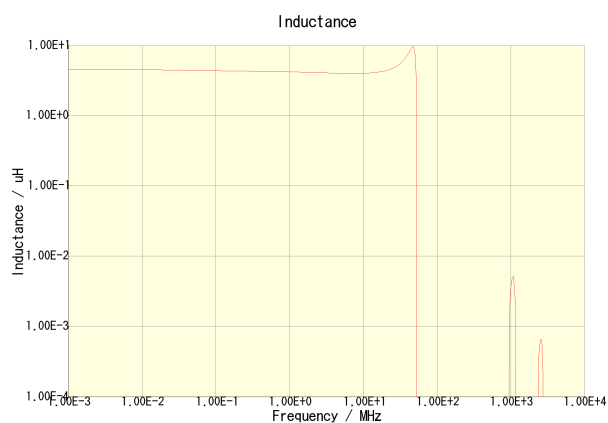
VLS3015ET-4R7M
