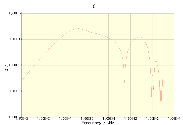
VLS3015ET-4R7M
