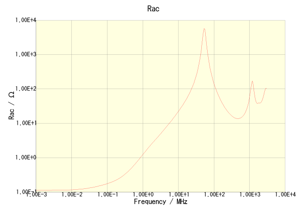
VLS3015ET-4R7M
