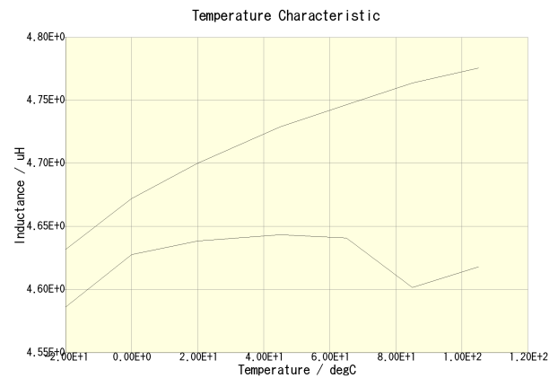
VLS3015ET-4R7M(DC = 0A)
