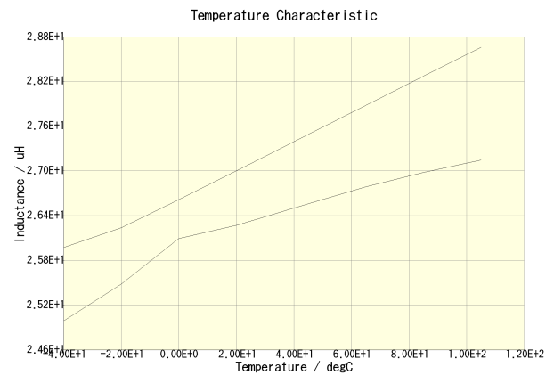
VLCF4020T-270MR48(DC = 0A)
