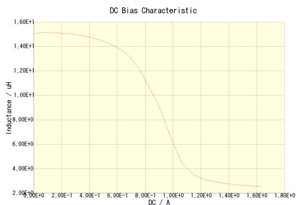
VLCF4018T-150MR59-2(Amb. Temp. = 20degc)
