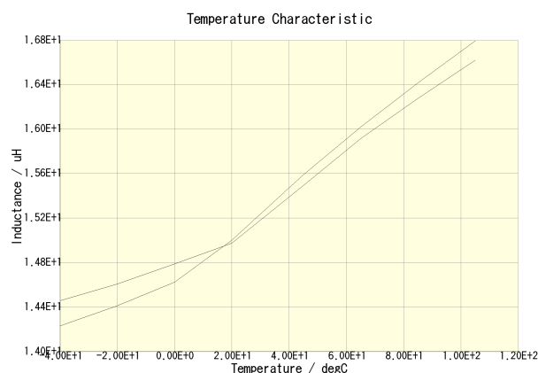
VLCF4018T-150MR59-2(DC = 0A)
