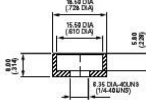
U825 (for cap U630)
