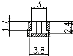
Section A-A' ACTUATOR
