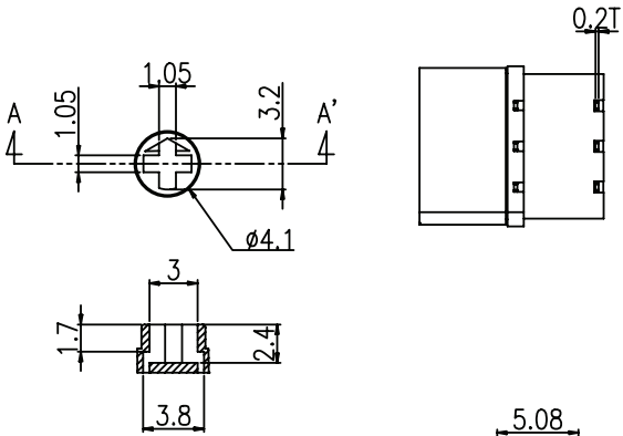
Section A-A' ACTUATOR
