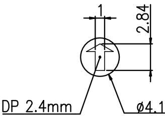
ACTUATOR
