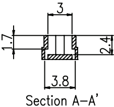
Section A-A' ACTUATOR
