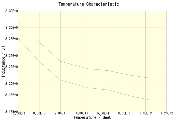
NLV32T-8R2J-PF(DC = 0A)
