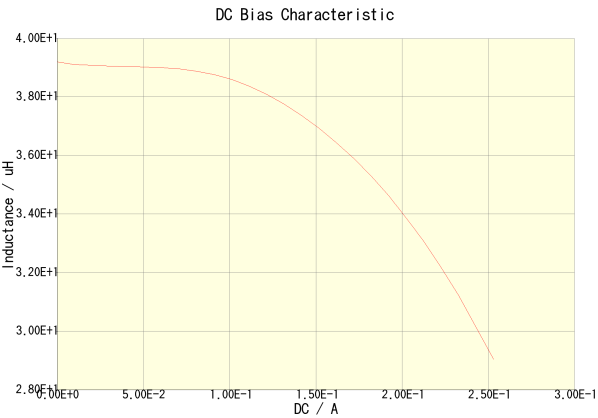
NLV32T-390J-PF(Amb. Temp. = 20degc)
