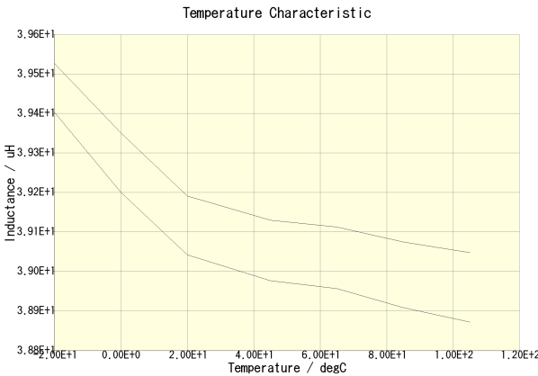
NLV32T-390J-PF(DC = 0A)
