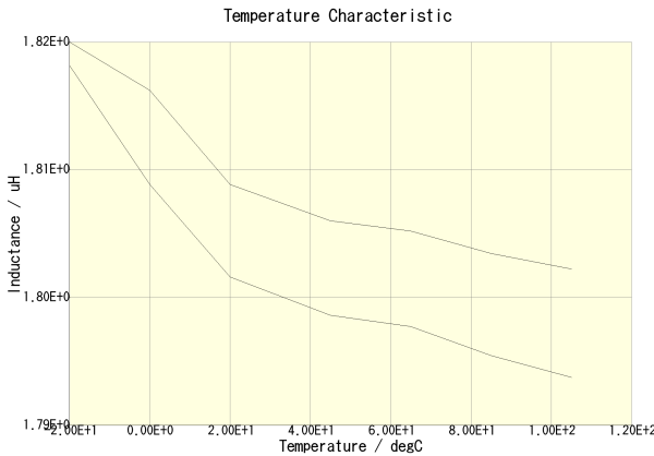
NLV32T-1R8J-PF(DC = 0A)
