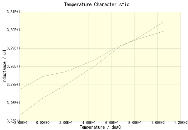
NLV25T-330J-PF(DC = 0A)
