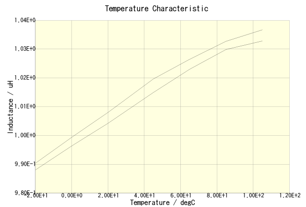
NLCV32T-1R0M-PF(DC = 0A)
