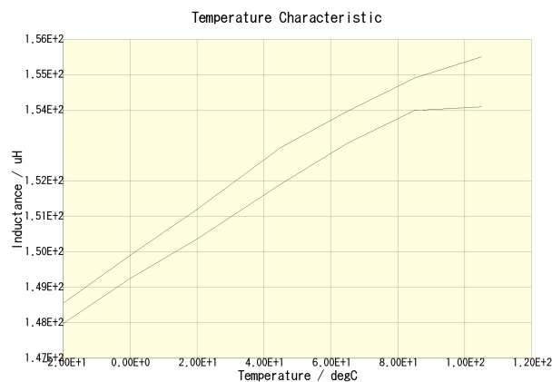
NLCV32T-151K-PF(DC = 0A)
