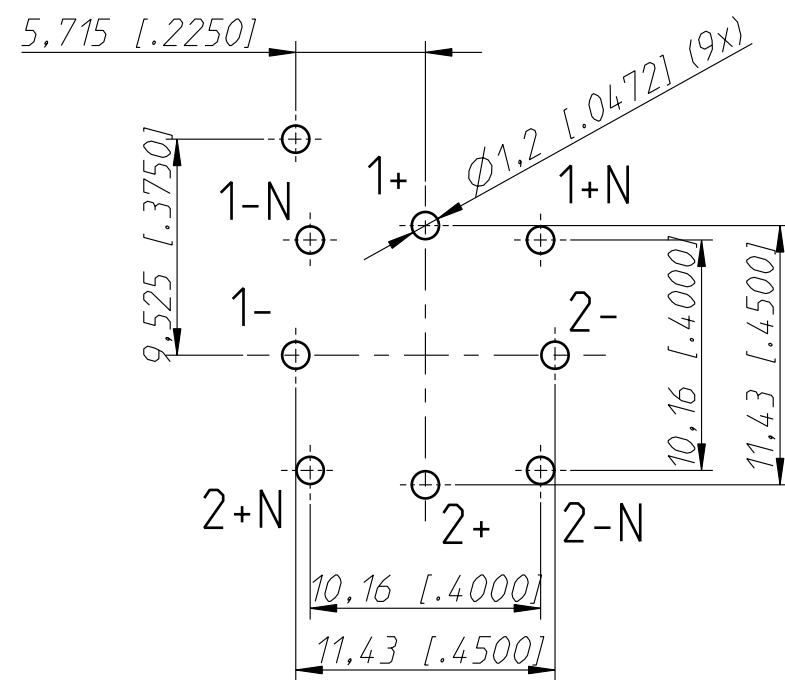
Printbohrplan (Bestückungsseite) PCB-Layer (Component Side)
