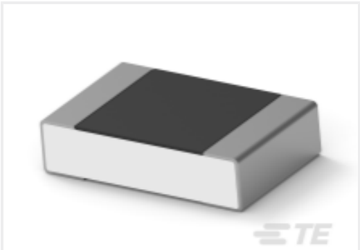
TE Part #9-2176376-5 RQ 0805 118K 0.1% 10PPM 1K RL
