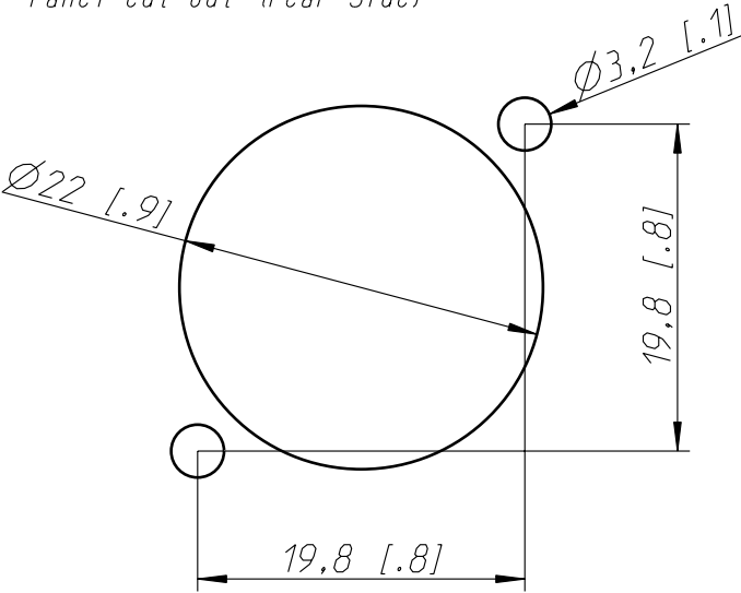
Frontplattenausschnitt (Rückseite) Panel cut out (rear side)
