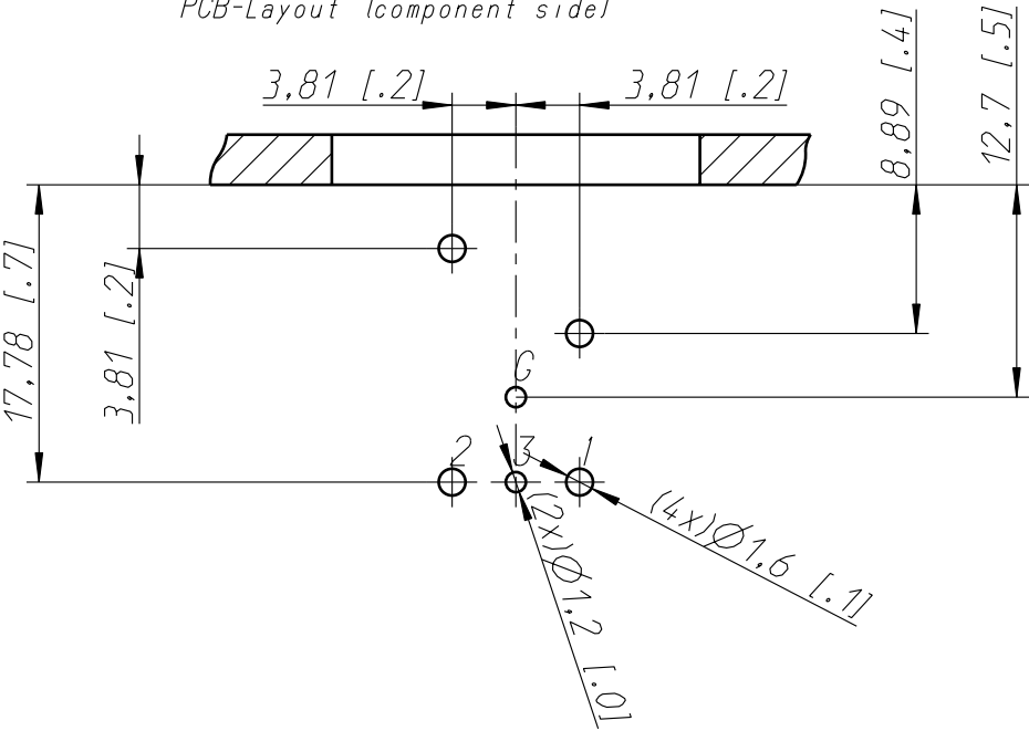
Print-Bohrplan (Bestückungsseite) PCB-Layout (component side)
