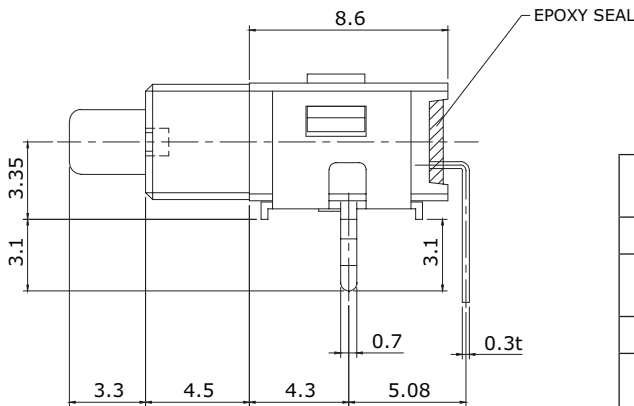
3.3 MM ACTUATOR
