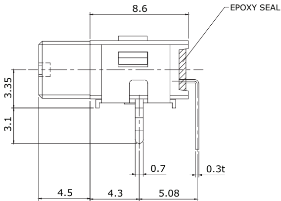
FLUSH ACTUATOR
