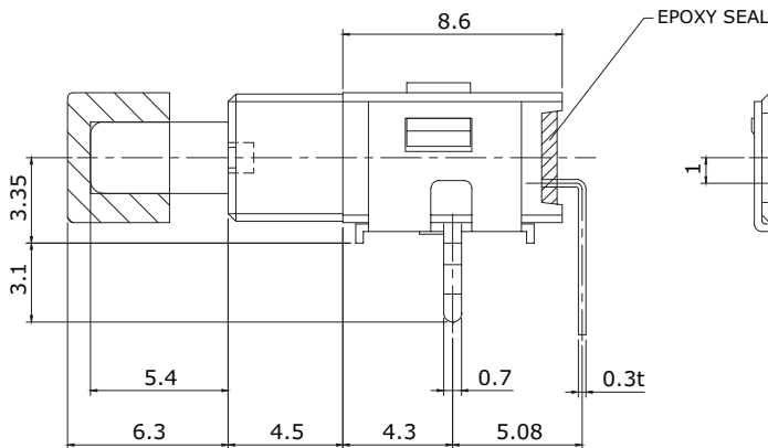
5.4 MM ACTUATOR
