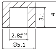
ACTUATOR CAP
