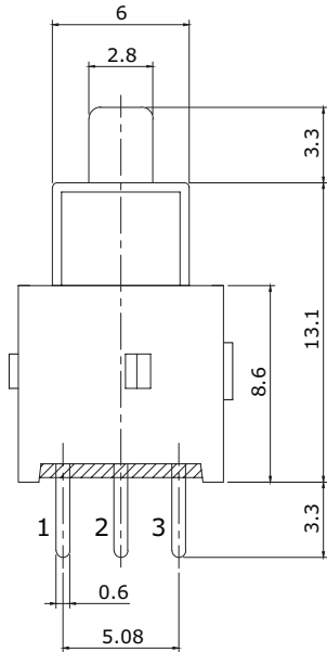
3.3 MM ACTUATOR
