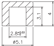
ACTUATOR CAP
