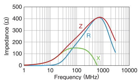
MMZ0402S241CT000
