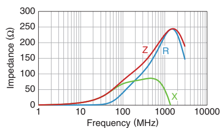
MMZ0402Y750CT000
