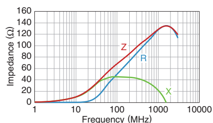
MMZ0402S700CT000
