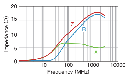
MMZ0402S100CT000
