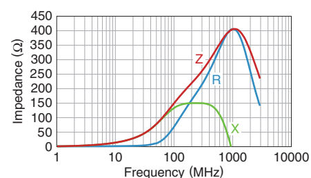
MMZ0402Y151CT000
