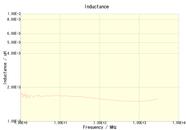
MLG1005S1N6ST000
