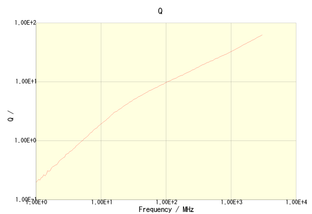
MLG1005S1N6ST000
