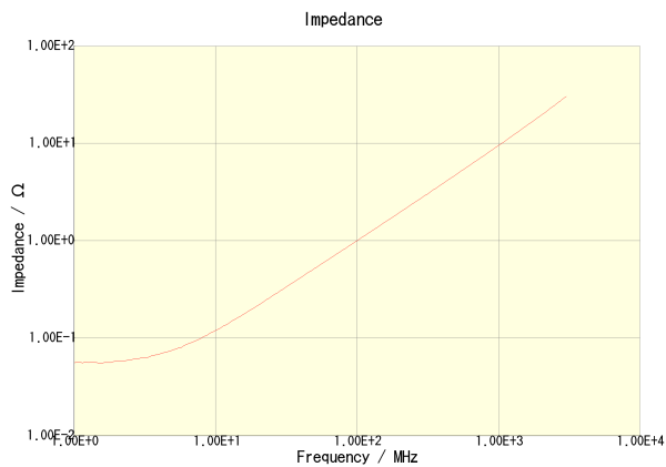
MLG1005S1N6ST000
