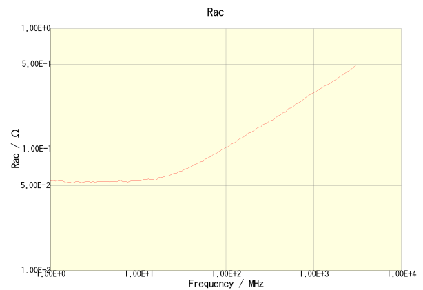
MLG1005S1N6ST000
