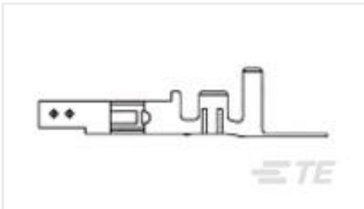
TE Part #1586317-3 VAL-U-LOK SKT PHBZ SN 26-22 LP
