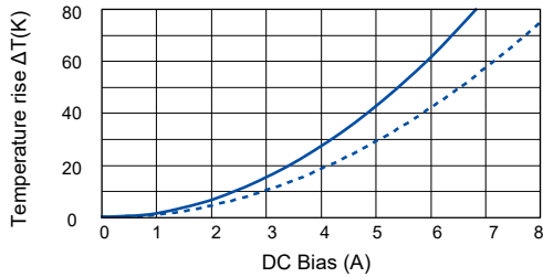
[ ETQP3M2R2YFP ]
