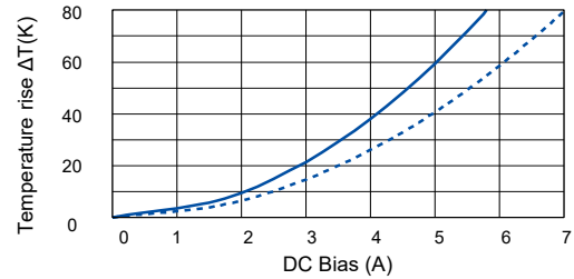
[ ETQP3M3R3YFP ]
