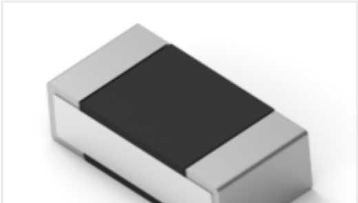
TE Part #7-2176311-5 RP 1E 0.1W 6K81 0.1% 25PPM 1K RL
