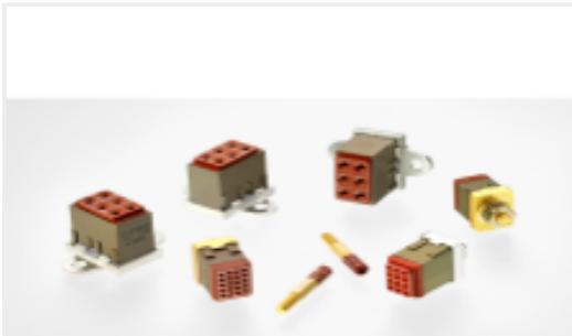
TE Part #CTJ722K01C-7067 MODULE ASSY
