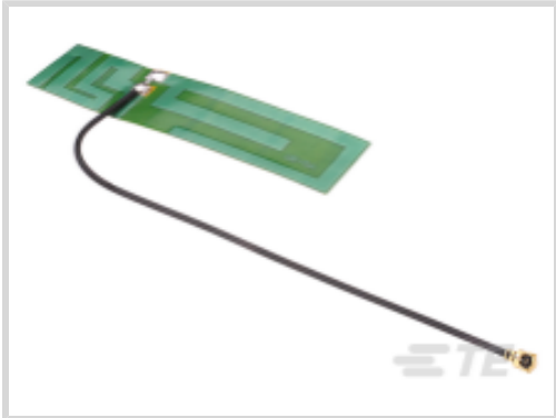
Antennas
