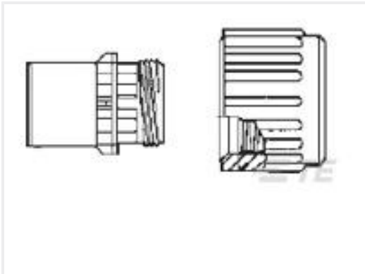
TE Part #213671-1 CPC 18-10 PLUG KIT W/CPLG RING
