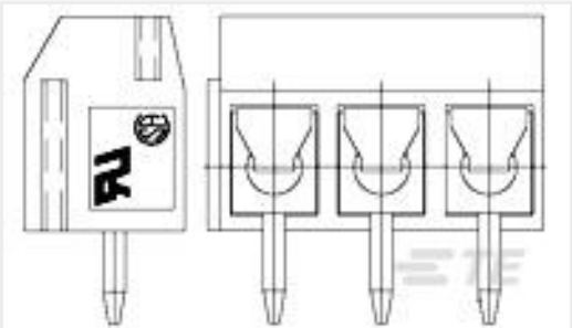
TE Part #1776244-3 3P TB ,90deg, VT, 5mm, Blue,w /interlock
