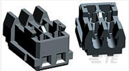
TE Part #1-353293-4 MINI CT MT REC ASSY 14P GRAY
