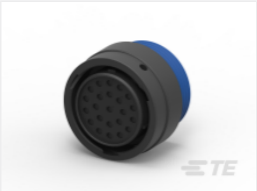
TE Part #YHDP26-24-23SEL024 PLG, 23P, BLK, E, WTHD, 16, S
