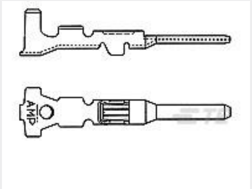
TE Part #282109-3 MINI MIC TAB CONTACT
