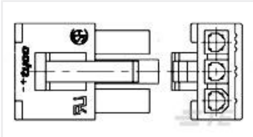
TE Part #1586106-3 3P RCPT VAL-U-LOK SR V0
