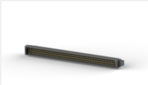
TE Part #5-1375583-8 09 MTE VERTICAL SMT HDR 30 AU
