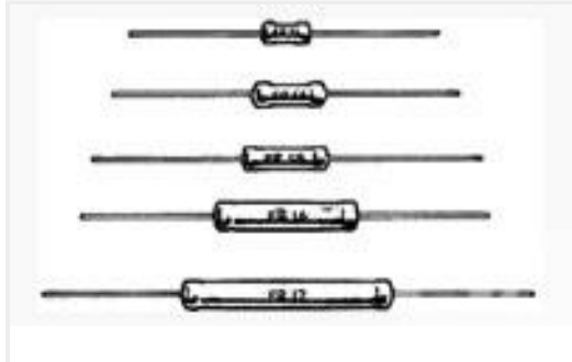
TE Part #4-1623746-8 ER74 6K8 5% AMMO PK
