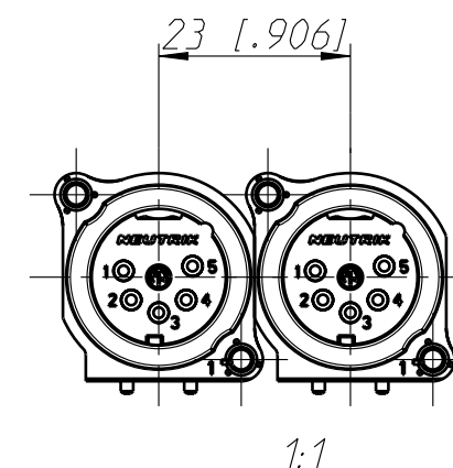
min. Einbauabstand min assembling distance
