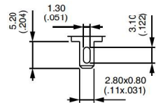
2 Solder lug
