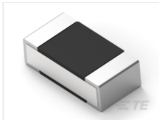
TE Part #2176308-6 RP 1E 0.1W 150K 0.1% 25PPM 5K RL
