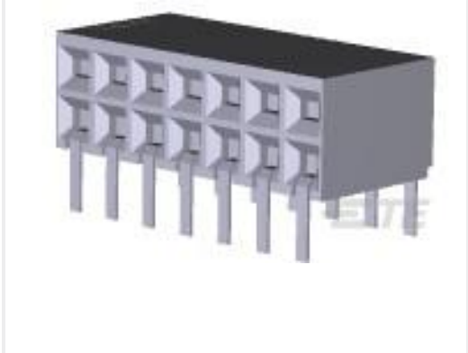
TE Part #1-5535512-7 14 MODII HORZ DR CE EESS .100
