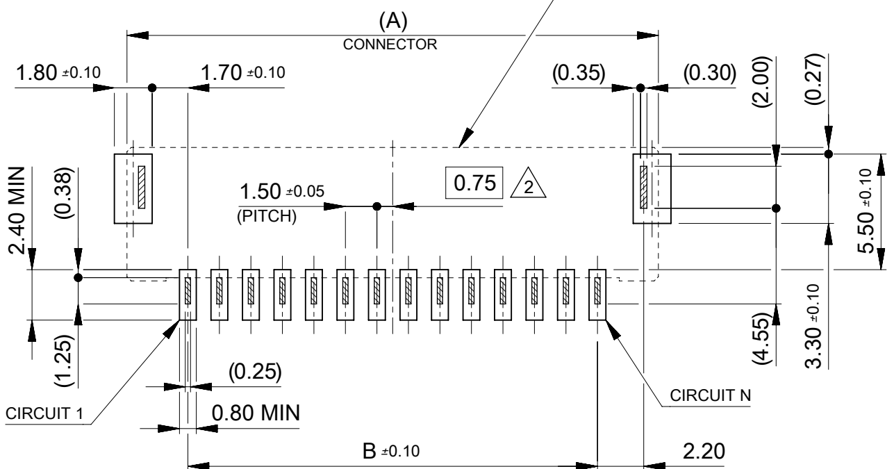
基板レイアウト(参考) PCB PATTERN LAYOUT (REFERENCE)
